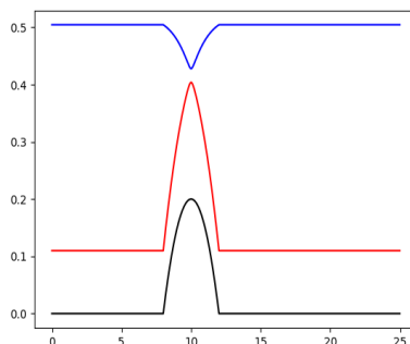
FIGURE 5.9 – Solutions stationnaires pour \beta = \beta_m + 0.001 et \alpha = 0.1 . Solution surcritique ( u > c ) en rouge et souscritique ( u < c ) en bleu. Le fond est en noir
