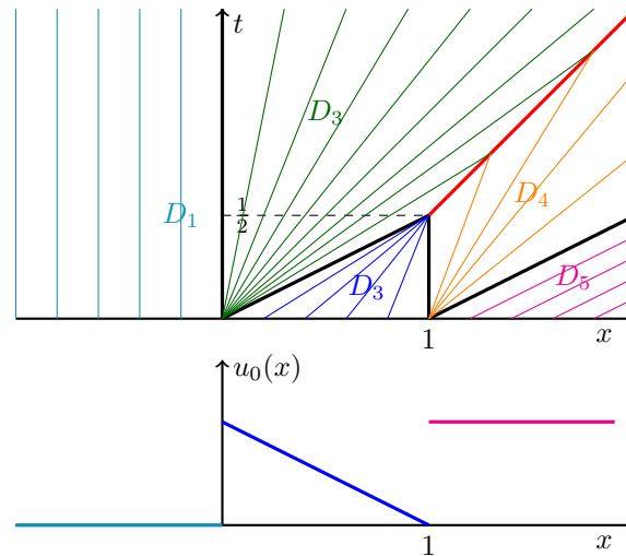
Figure 5.6: 5.6 - En haut : Droites caractéristiques pour l'équation de Burgers avec condition initiale u_0 ; en rouge la ligne de choc, en noir les lignes de discontinuité C^1 – En bas : allure de la condition initiale u_0 .
