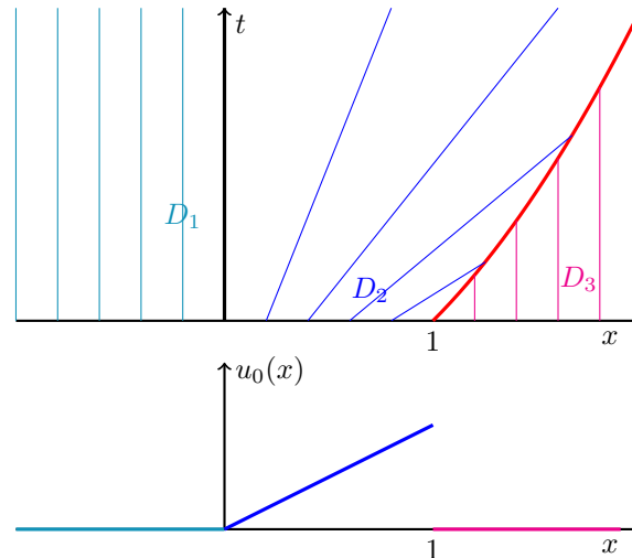
Figure 5.7: En haut : Droites caractéristiques pour l'équation de Burgers avec condition initiale u_0 ; en rouge la ligne de choc, en noir les lignes de discontinuité C^1 – En bas : allure de la condition initiale u_0 .
