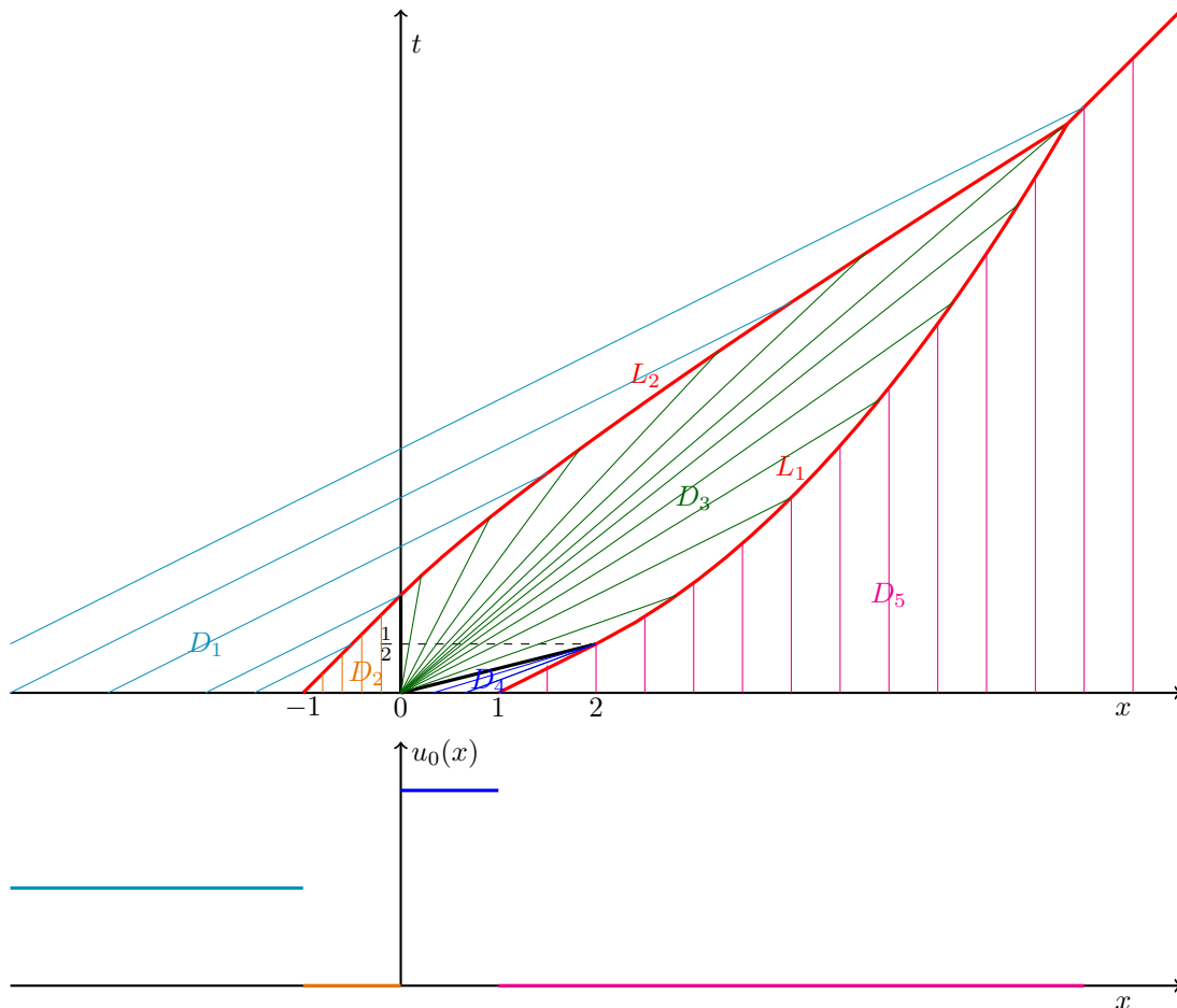
Figure 5.8: En haut : Droites caractéristiques pour l'équation de Burgers avec condition initiale u_0 ; en rouge la ligne de choc, en noir les lignes de discontinuité C^1 – En bas : allure de la condition initiale u_0 .
