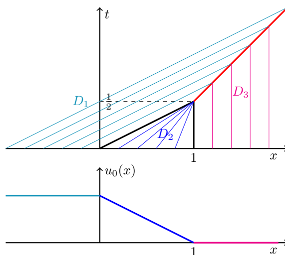
Figure 5.5: Exercice 5.4 page 225. En haut : Droites caractéristiques pour l'équation de Burgers avec condition initiale (5.50) En rouge la ligne de choc, en noir les lignes de discontinuité C^1 . – En bas : allure de la condition initiale u_0 .
