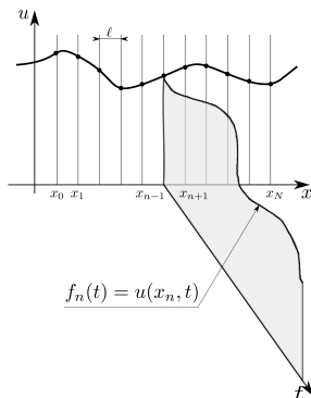
FIGURE 8.1. – Schéma de différences finies : la fonction u(x, t) est échantillonnée aux points x_n = n\ell de l'espace ; Si les fonctions f_n(t) = u(x_n, t) peuvent être calculées, nous disposons alors d'une bonne approximation de la fonction u(x, t) .
