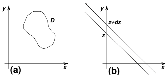
FIGURE 2.1. – (a) La probabilité pour qu’une mesure combiné (x, y) tombe dans un domaine \mathcal{D} est \int \int_{\mathcal{D}} p(x, y) dx dy . (b) Pour que la variable aléatoire Z = X + Y tombe dans le domaine [z, z + dz] , il faut que le résultat (x, y) d’une mesure combinée tombe dans le domaine délimitée par les deux droites ;
