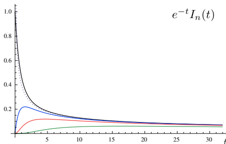
FIGURE 4.3. – Les fonctions de Bessel e^{-t}I_n(t) pour n = 0 (noir), n = 1 (bleu), n = 2 (rouge) et n = 4 (vert). La courbe en pointillé est la fonction 1/\sqrt{2\pi t} qui est la limite asymptotique de toutes ces fonctions, et reflète leur décroissance lente en fonction de t .
