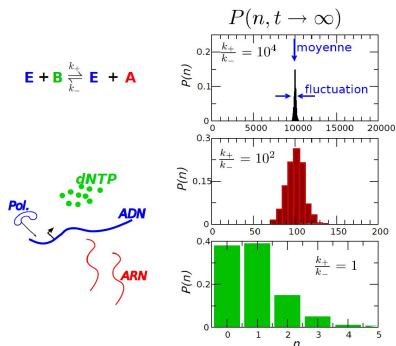
FIGURE 4.1. – Transcription d’ARN. Dans la réaction chimique ci-dessus, E représente l’ADN et le polymérase (en bleu), B les dNTP (en vert) et A l’ARN (rouge). Quand le nombre de molécules est important (cas k_+/k_- = 10^4 ), les fluctuations sont faibles et la dynamique peut se traiter par des équations déterministes. Quand par contre le nombre moyen de molécule d’ARN est faible ( k_+/k_- \approx 1 ), le système doit se traiter par les probabilités.
